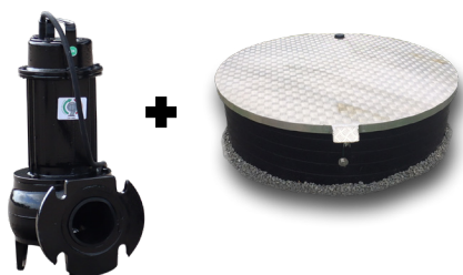
3" Pumpe 0,9 kW - 16 l/sek
